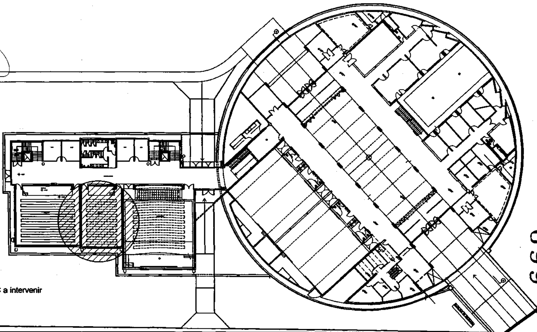
PLANO DE UBICACIÓN PLANTA BAJA
