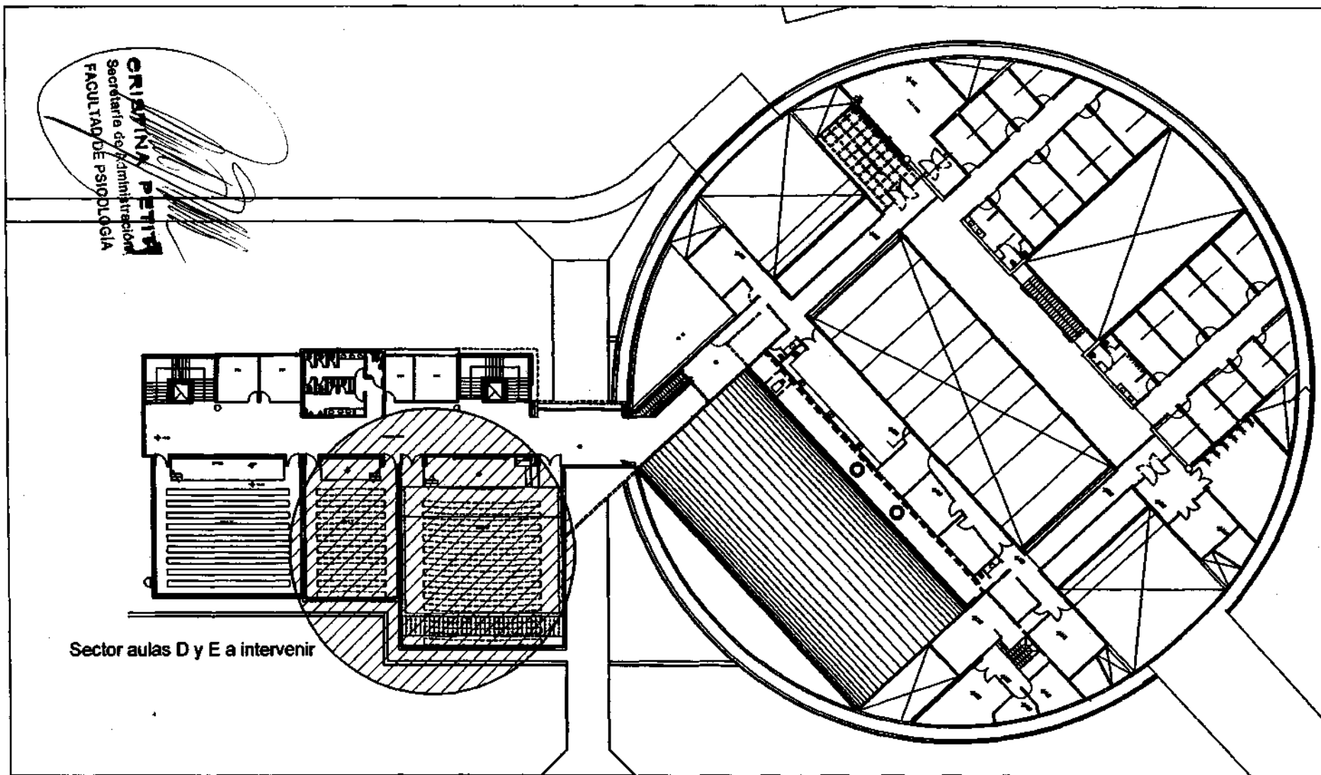
PLANO DE UBICACIÓN PLANTA PRIMER PISO
