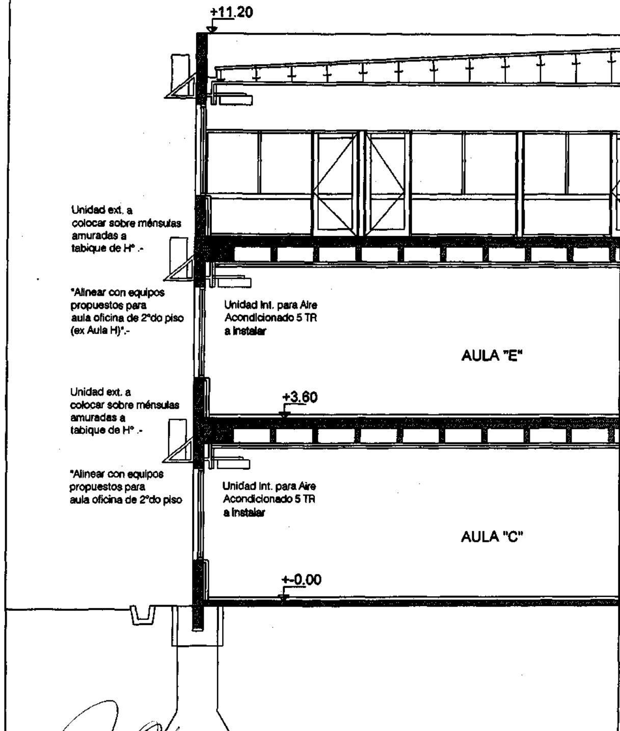
CORTE ESQUEMÁTICO DE COLOCACIÓN DE EQUIPOS esc 1:125
