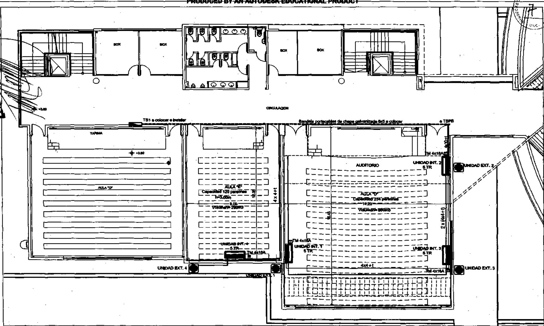
EQUIPOS A* A* EN AULAS "D", "E" - PLANTA PRIMER PISO Esc 1:125
