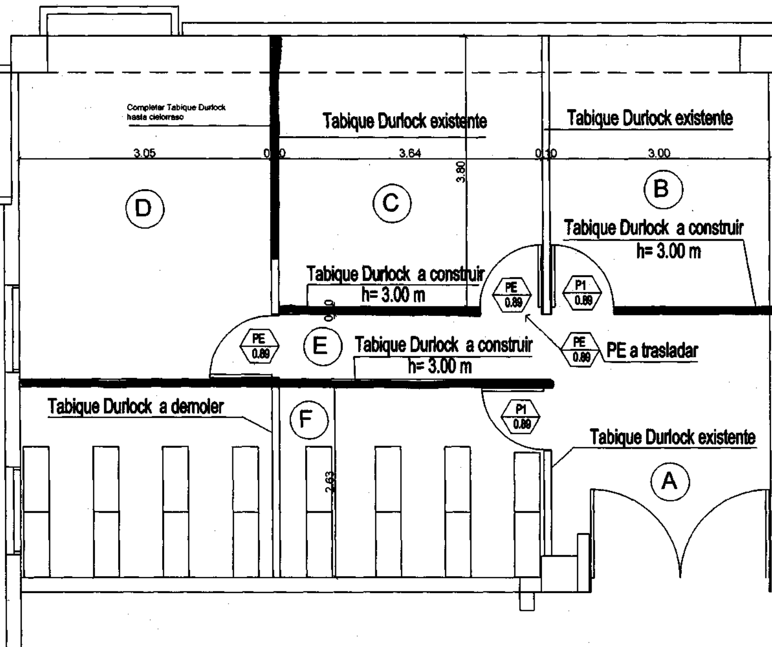
PLANTA TABIQUERÍA DURLOCK
